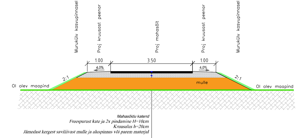
Mahasõidu ristlõige 1:100
